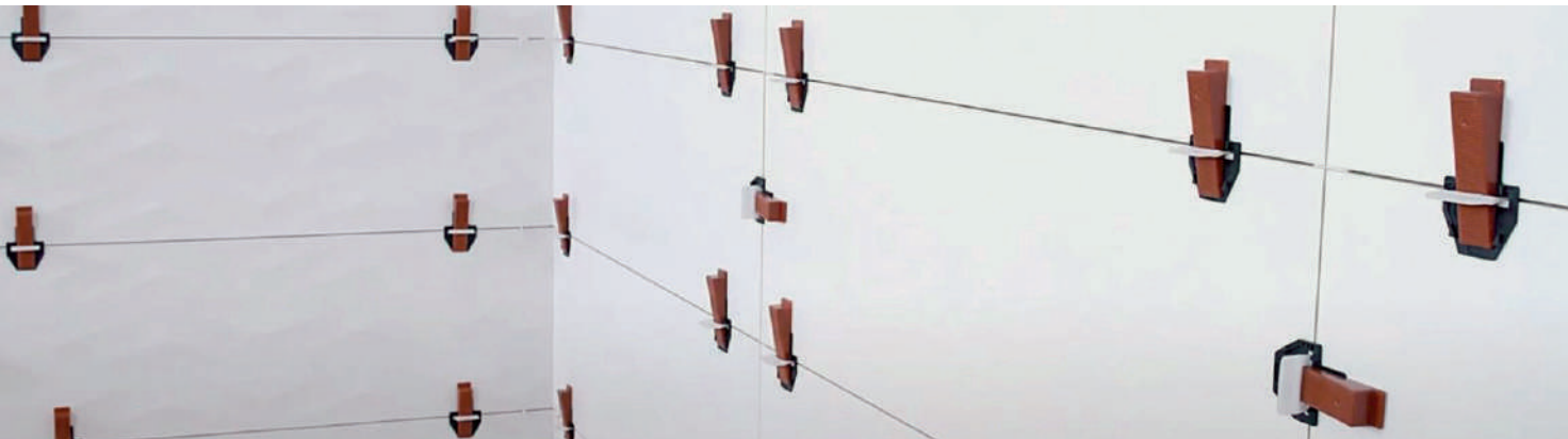
Example of using the RLS Levelling System to lay tiles on walls and floors. Exemple de pose R.S.L.-Système nivelant Raimondi dans les faïences et les carreaux de sol.
